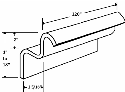
DOOR REAR EDGE - 10' Part # 6086
