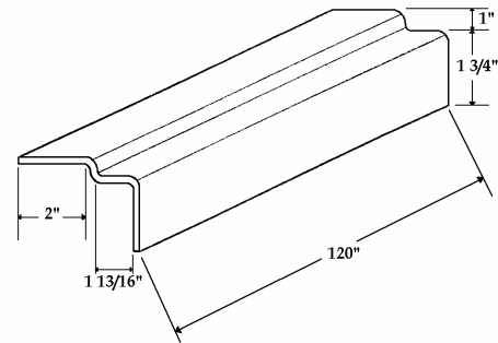
DOOR TOP RETAINER - 10' Part # 6088
