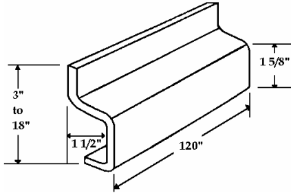
DOOR FRONT EDGE - 10' Part # 6082
