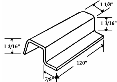
DOOR STOP - 10' Part # 6085
